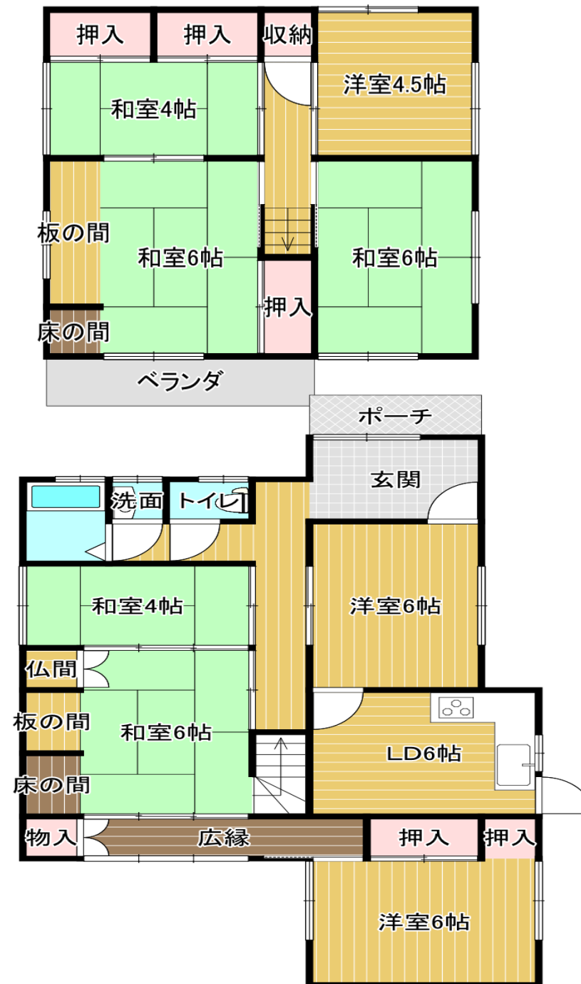
1・2階平面図
